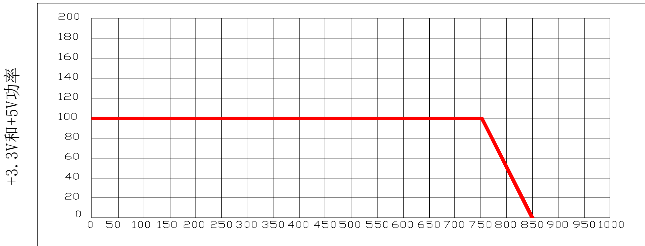
+12V 功率 (交叉负载)
